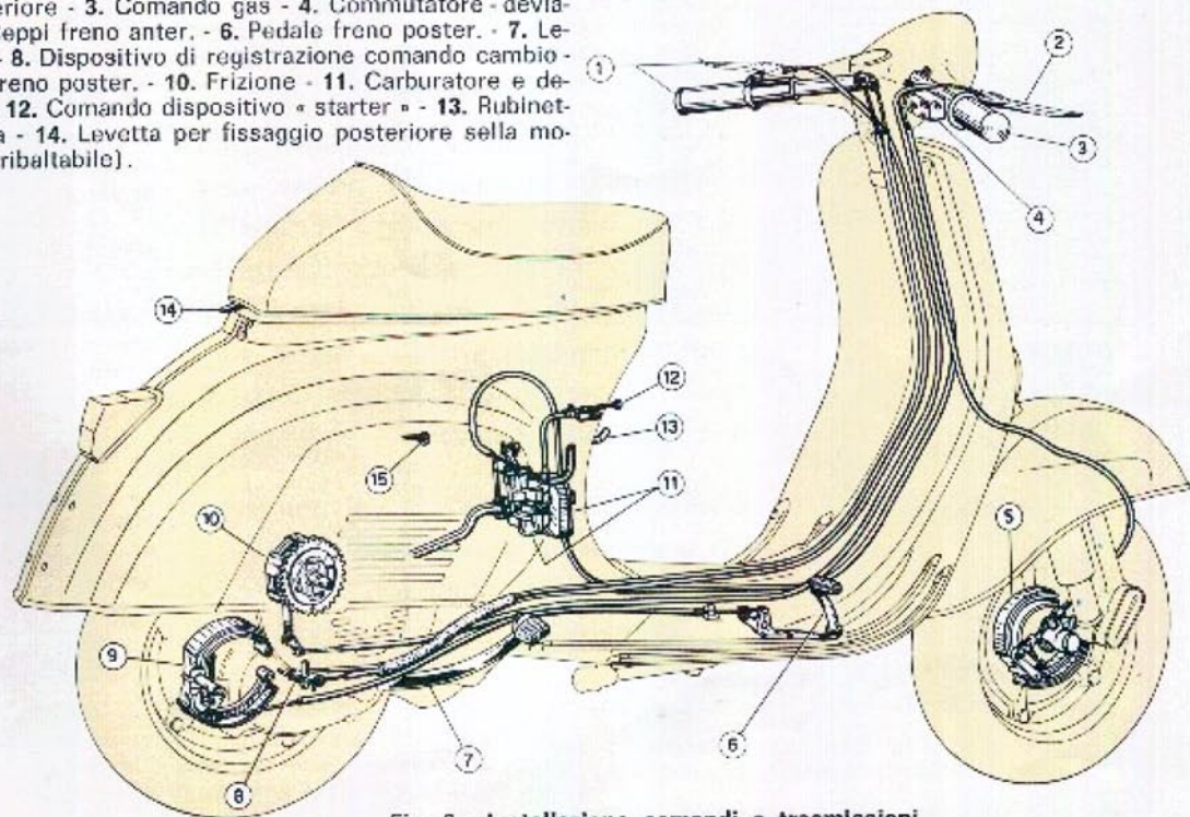
Fig. 2 - Installazione comandi e trasmissioni
