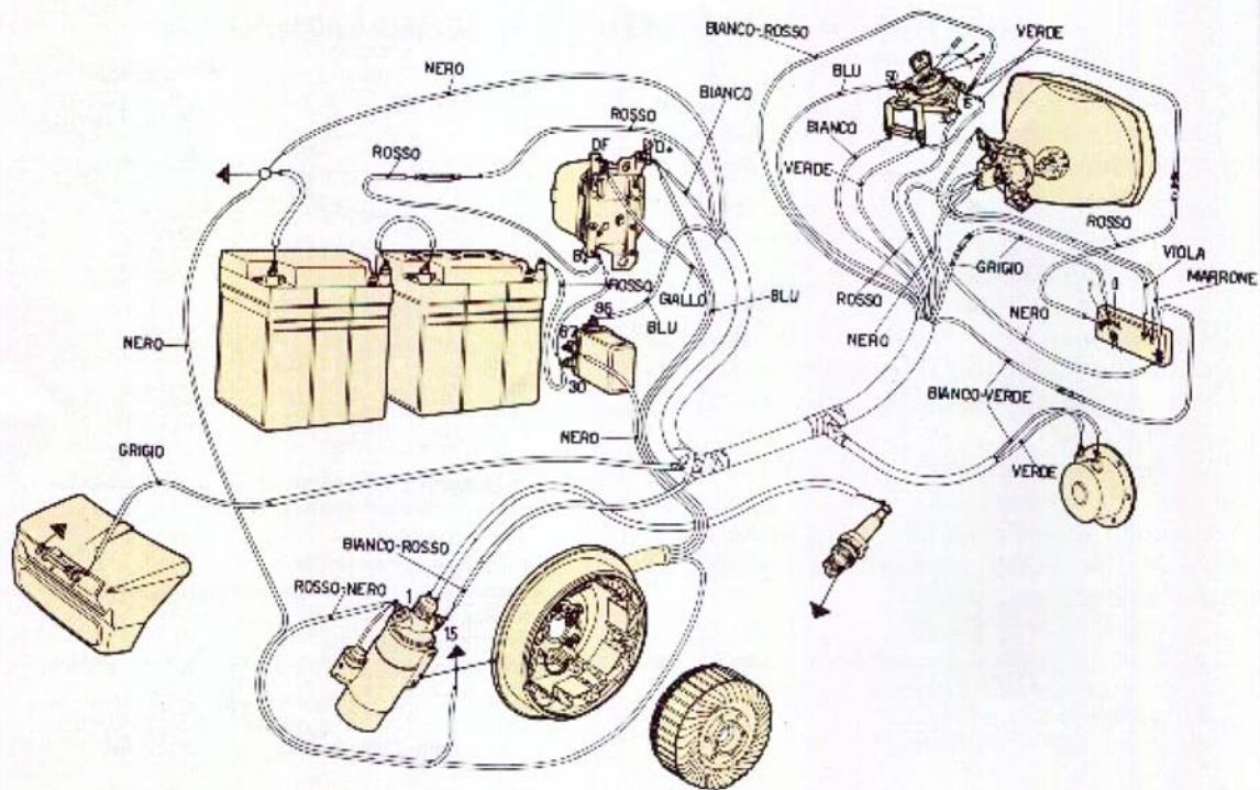
Fig. 28 - Schema installazione impianto elettrico
