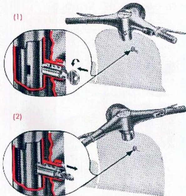
Fig. 3 - Serratura antifurto
