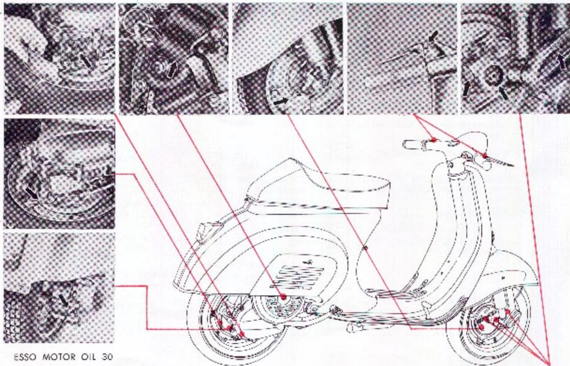
Fig. 17 - Schema della lubrificazione
