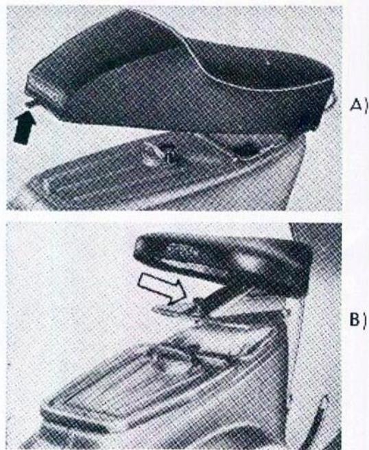
Fig. 4 - Ribaltamento sella allungata (« A ») e normale, a sbalzo, (« B »).
