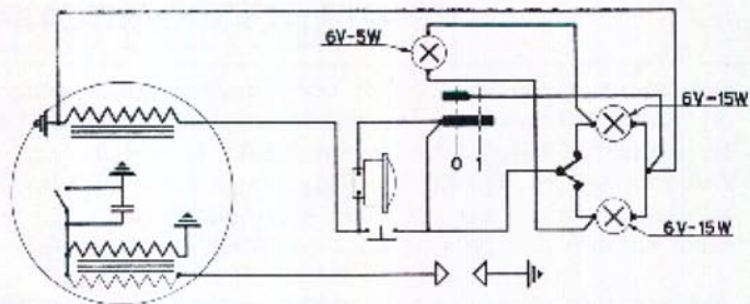
Fig. 21 - Schema dei collegamenti elettrici della Vespa 50.
