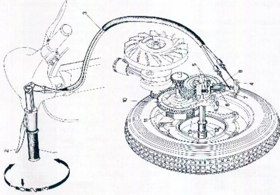
Fig. 7 - Schema del cambio
