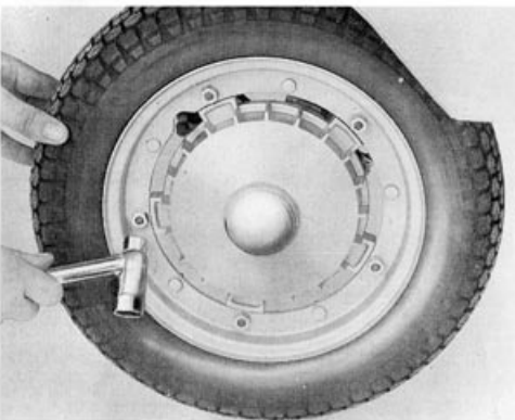
Fig. sopra: smontaggio ruota anteriore; per la ruota posteriore procedere in modo analogo.
