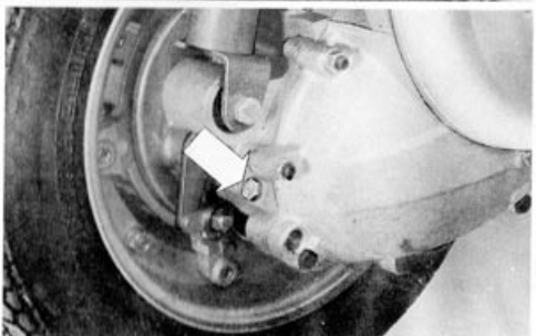
Fig. a destra in alto: foro di scarico dell'olio del cambio.
