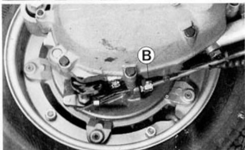
Fig. a destra in alto: A - Registro freno anteriore
